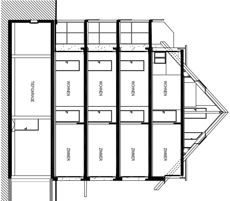
QUERSCHNITT
