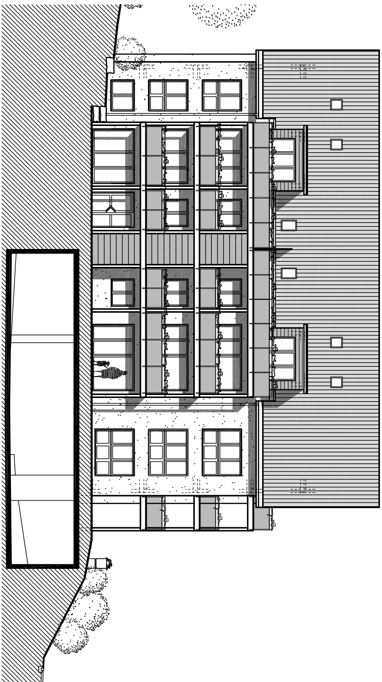
SÜDOST-FASSADE
